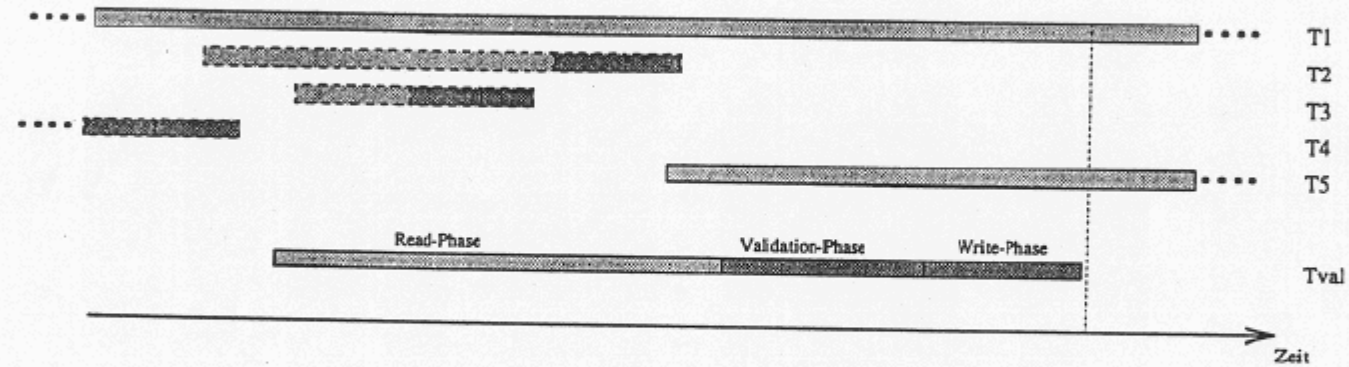
Abbildung 8: Vorwärtsvalidierung (FoC)
